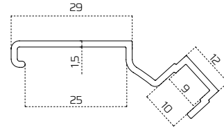
Küpeşte Uzatma Profili / Gunwale Extension Profile
