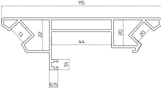
Küpeşte Profili / Gunwale Profile
