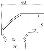
GeniŐ   Çıta Profili / Wide Internal Slat Profile
