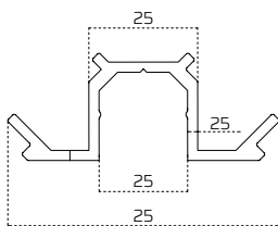
Köşe Dikme Kapak Profili / Corner Sewing Cover Profile
