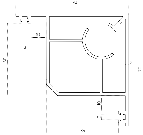
Küpeşte Köşe Profili / Gunwale Corner Profile
