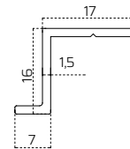
Küpeşte Kapak Profili / Gunwale Cover Profile 0,091 Kg/m
